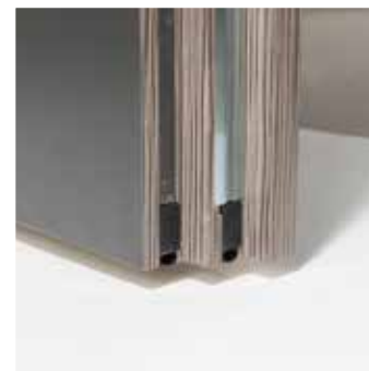
Zdvojený zvukově izolační padací práh
